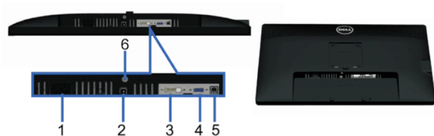
底部図
